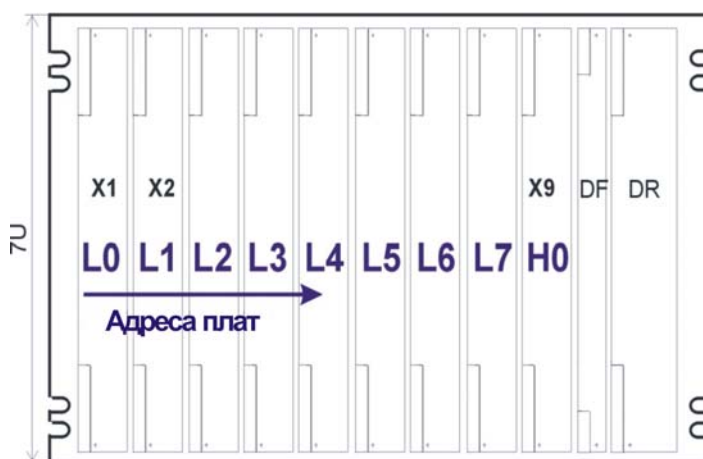
Рис. 3.4. ALFA-ERACK-KR с установленными платами (вид спереди).
